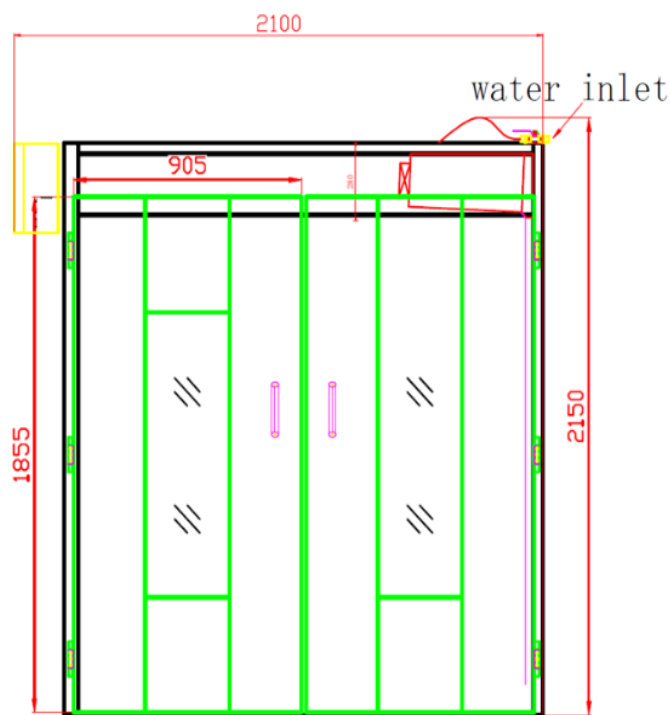
Габаритный чертеж MIRATEK PRF-2 (2 тележки 600х800)
